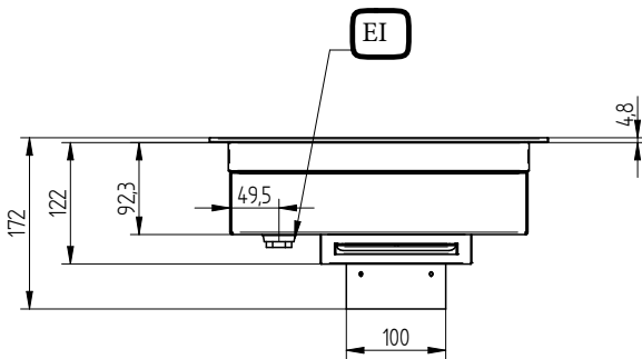
Alzado
